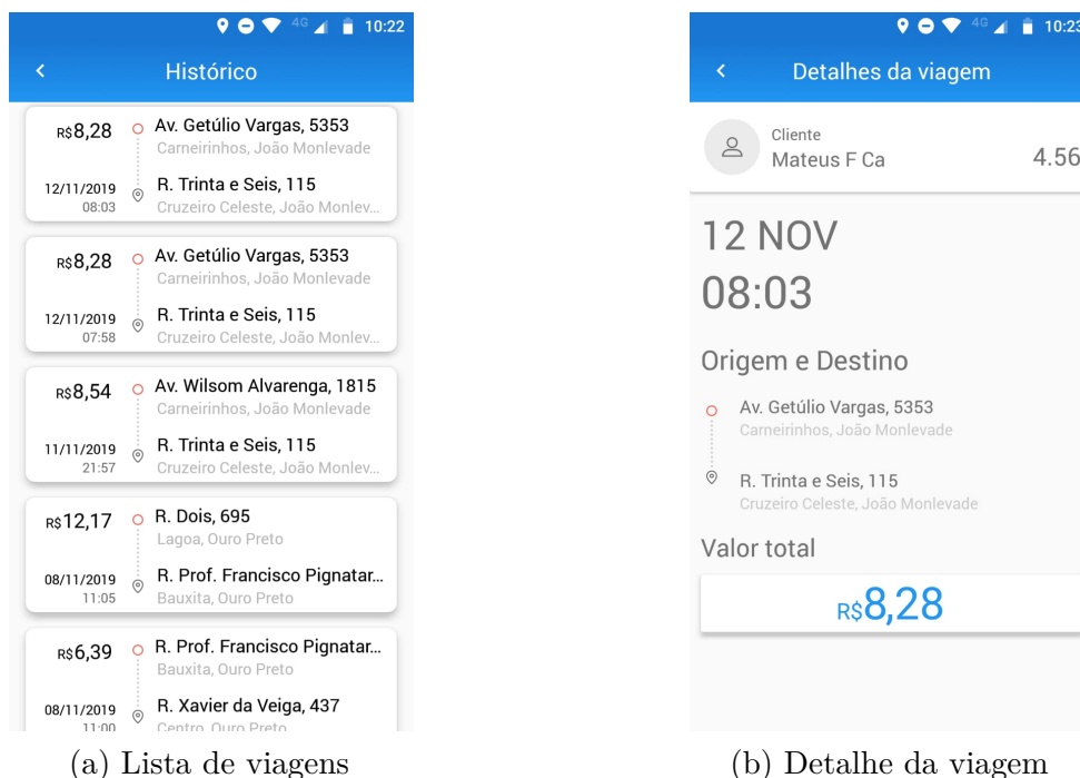
Figura 20 – Histórico
