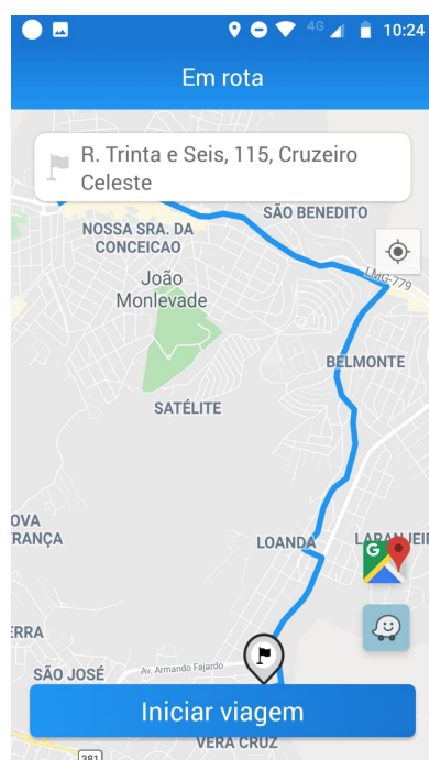
Figura 25 – Iniciar corrida
