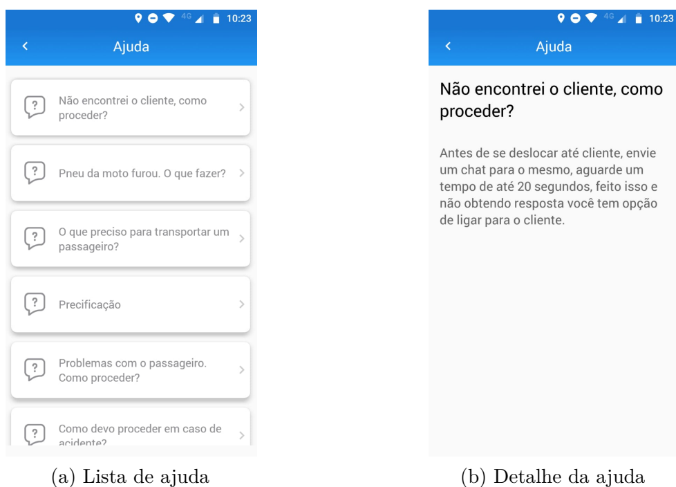
Figura 22 – Ajuda
