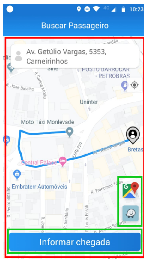
Figura 3 – Fragmentos
