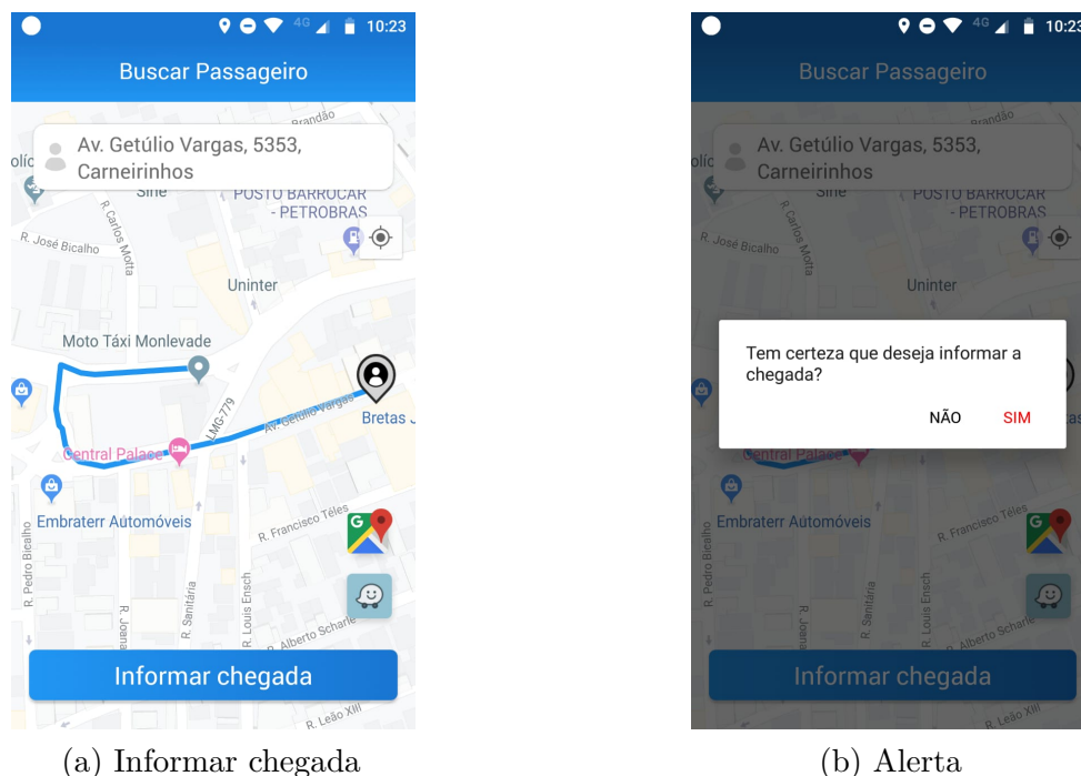
Figura 24 – Informar chegada
