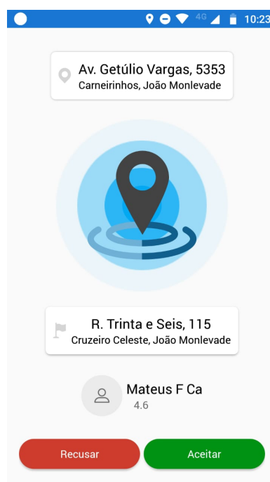
Figura 23 – Nova corrida
