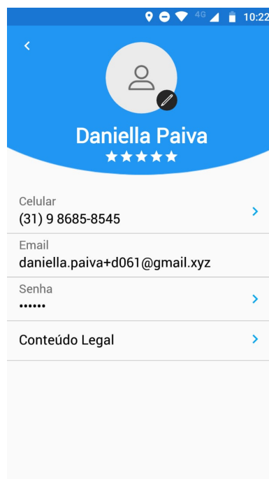
Figura 19 – Perfil
