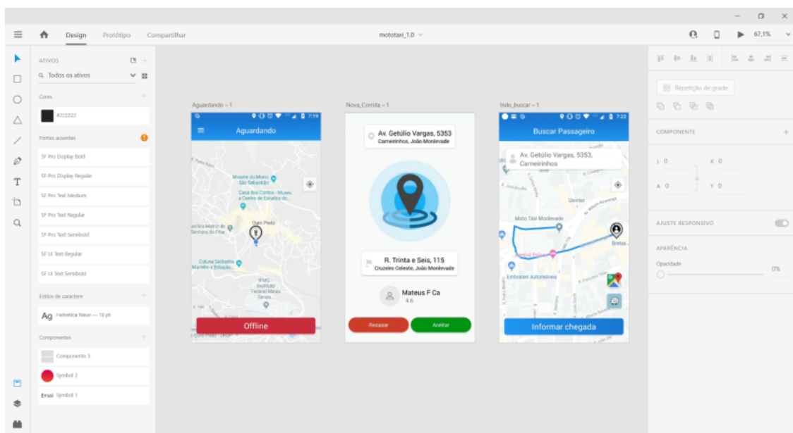
Figura 18 – Protótipos
