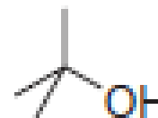
2-Metil-2-propanol (Álcool terc -butílico), um álcool 3°
