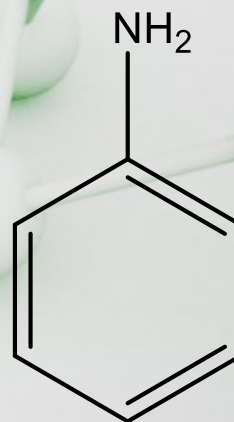
anilina
