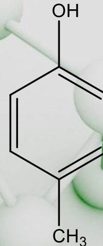
p -metilfenol
