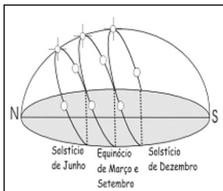
Figura 7. Movimento diário do Sol em uma localidade do hemisfério Sul.
